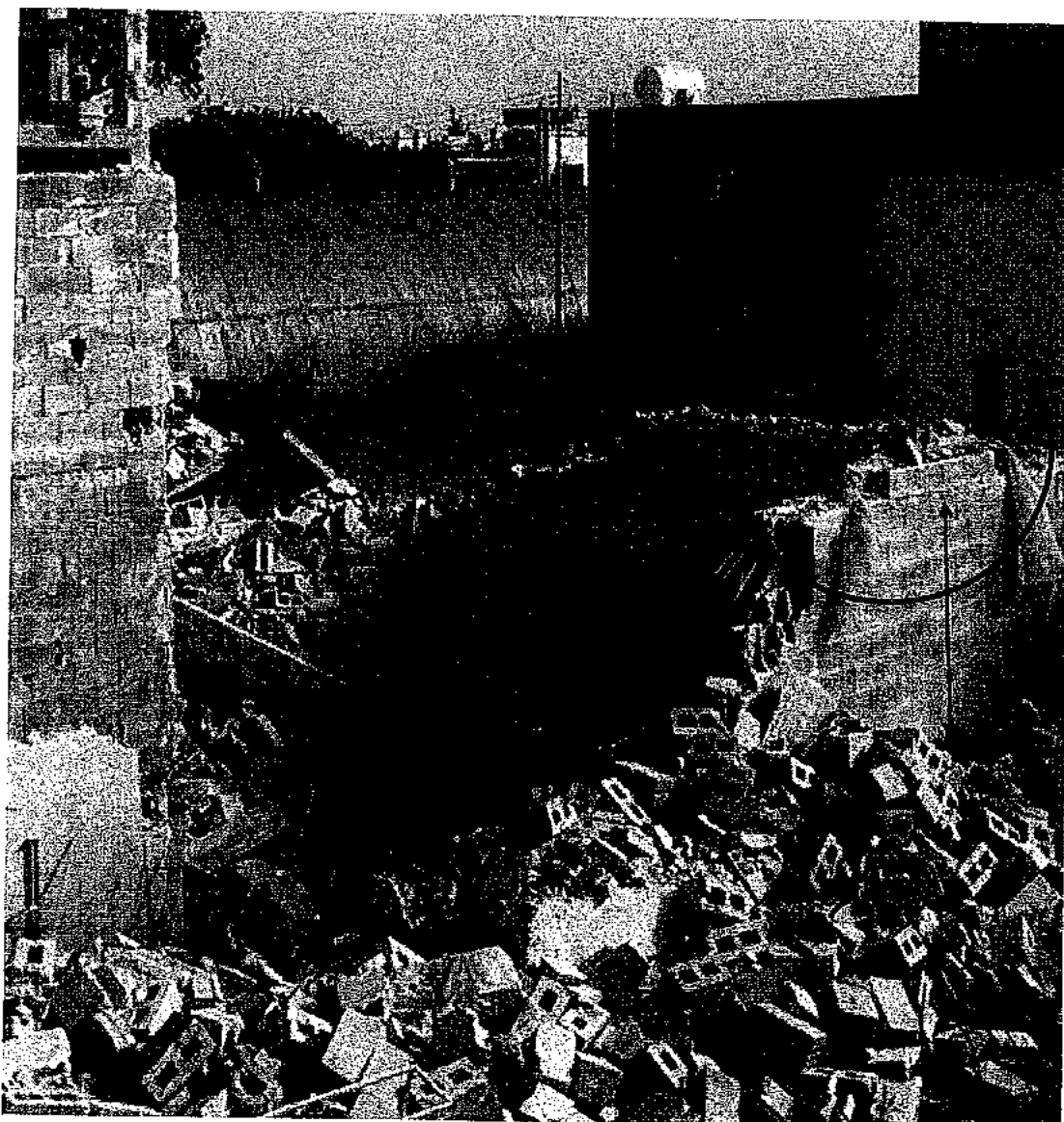
Dok. 38 Ritratt li juri l-għoli mill-qatran sal-filata li daret meta seħħ il-kollass (ċirku aħmar) u, fuq wara, il-briks maqsum min-nofs bħala riżultat tal-kollass tal-planki, (vlegġa hamra).
