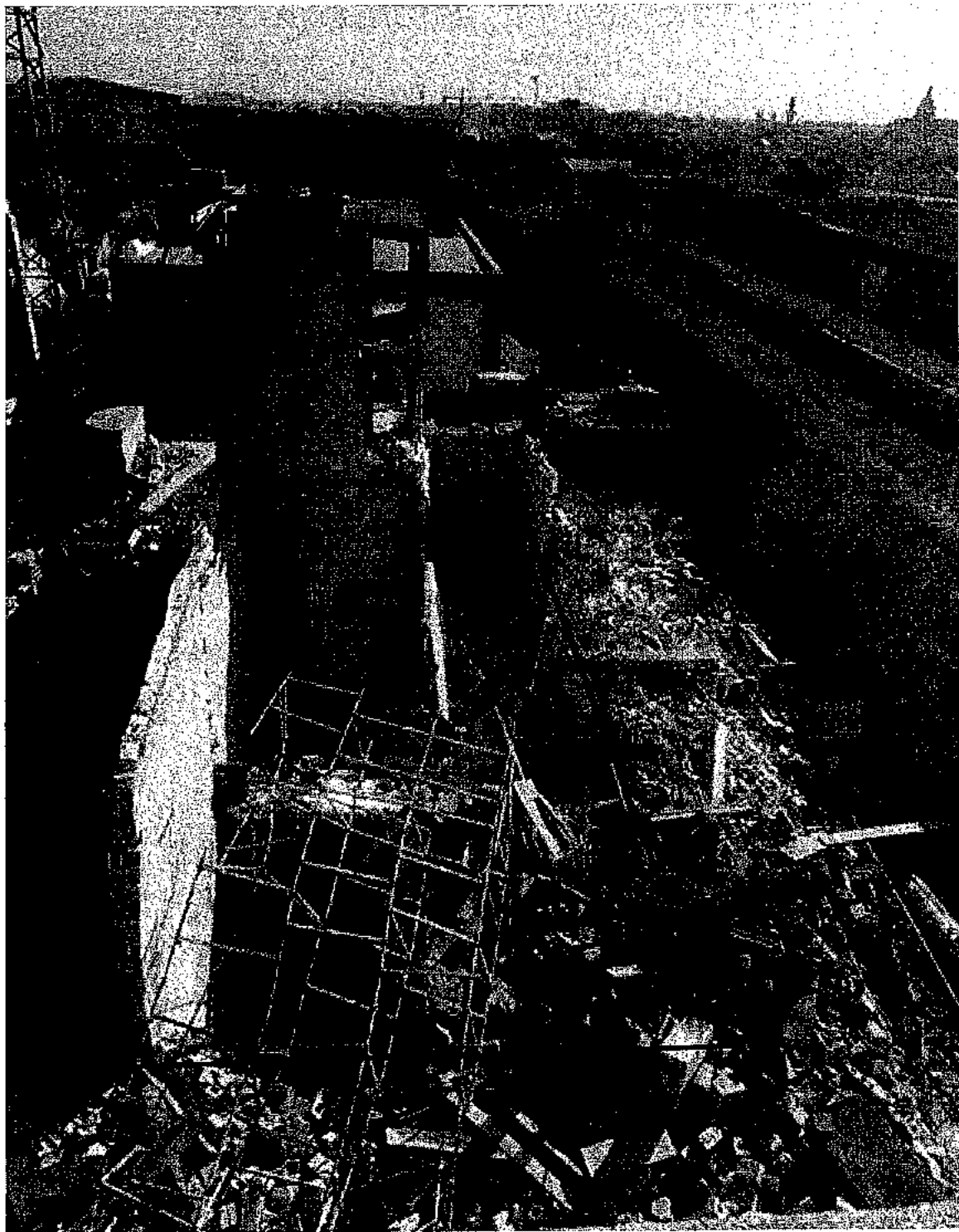
Dok. 35 Ritratt meħud mill-bejt tal-fabbrika Garcia Woodworks – ċ-ċirku bl-aħmar juri nuqqas ta' mursaljar bejn il-ħajt ta' barra u d-diviżorji
